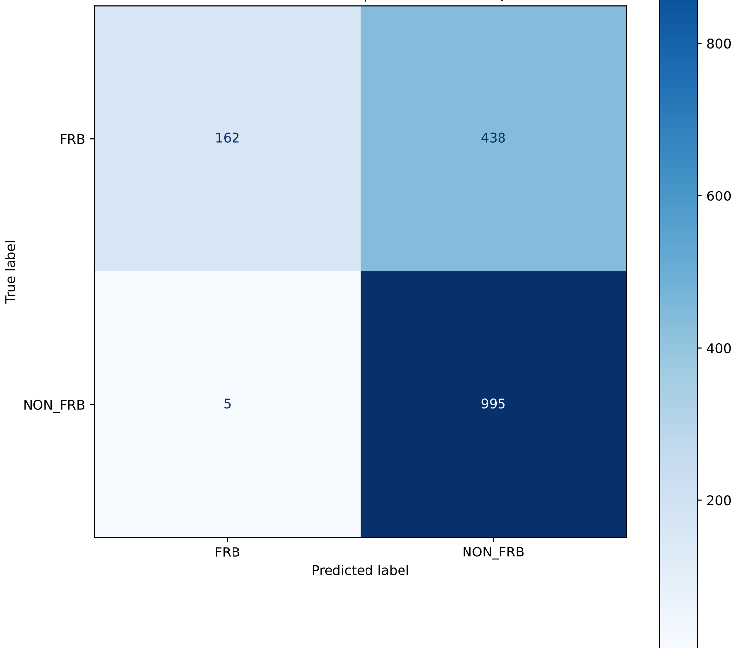
Matriz de Confusao Linhas: classe verdadeira | Colunas: classe prevista
