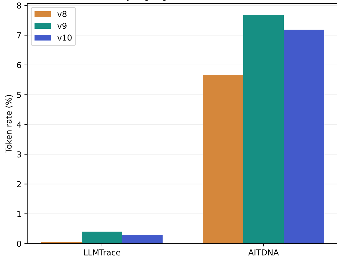
Human tokens falsely highlighted
