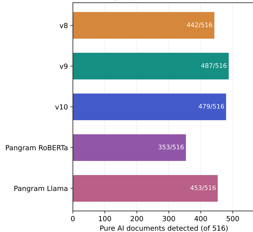
LLMTrace pure AI
