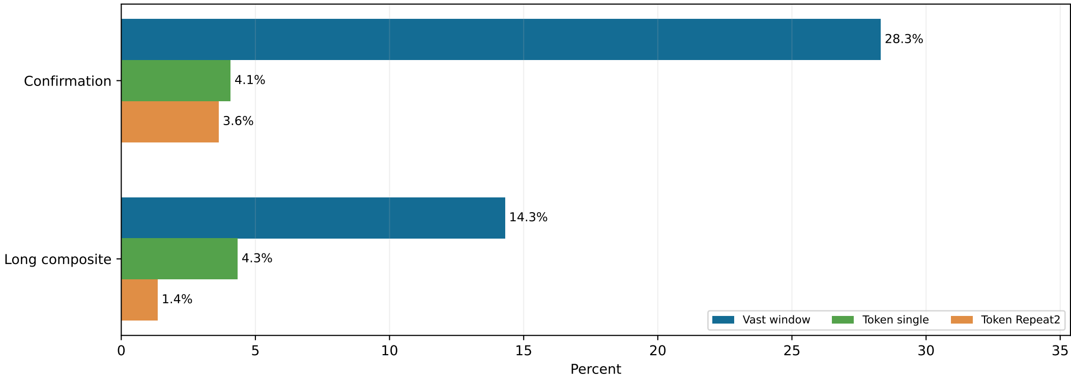
AI token recall
