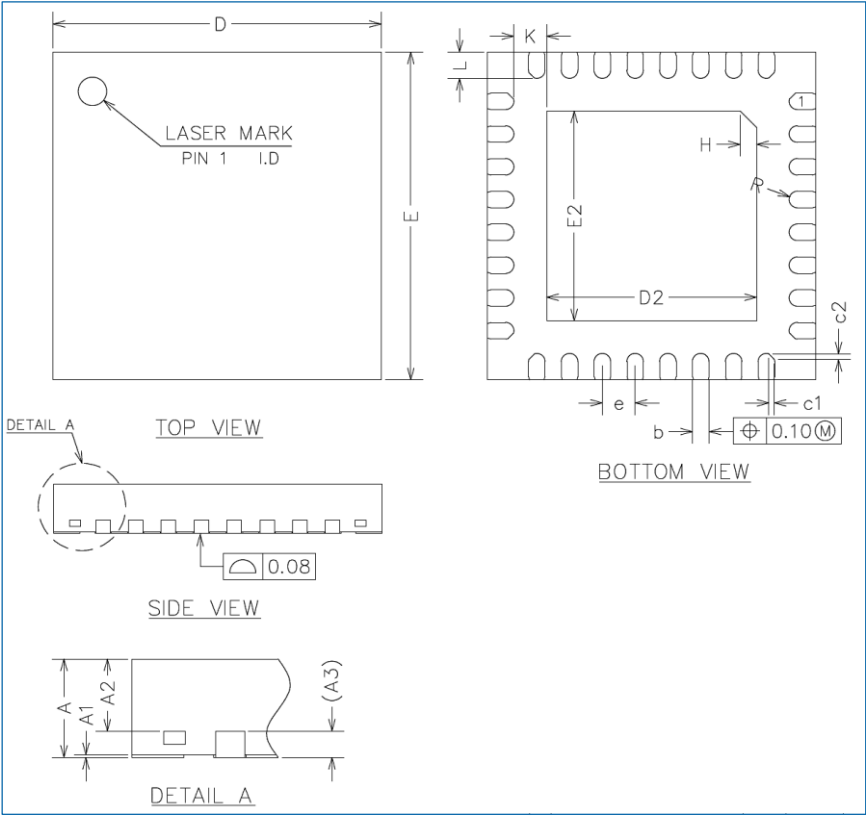
图 7-4 QFN32 封装尺寸图
