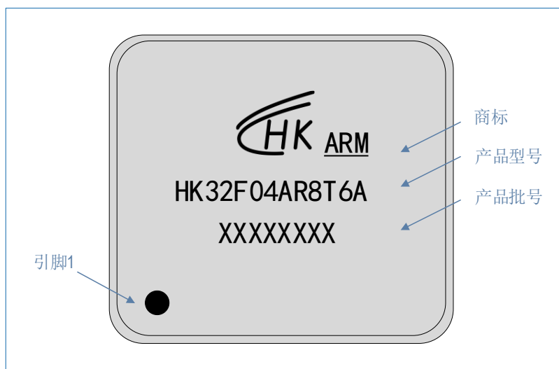
图 7-8 LQFP64 HK32F04AR8T6A 丝印示例
