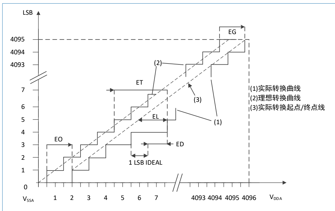
图 4-3 ADC 精度特征
