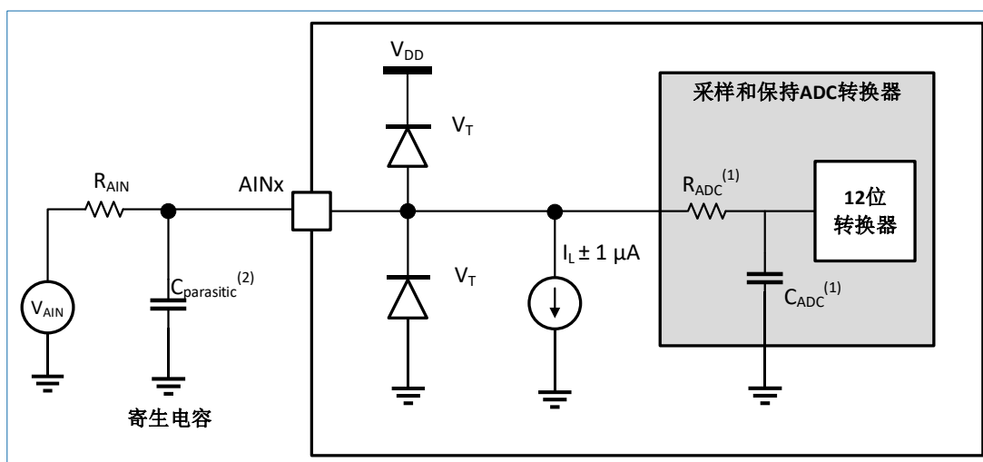
图 4-4 ADC 的典型连接图
