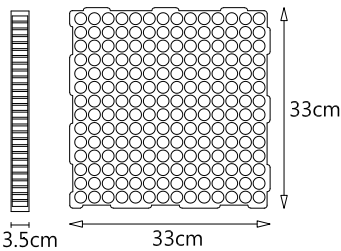
雙面過濾排水板
