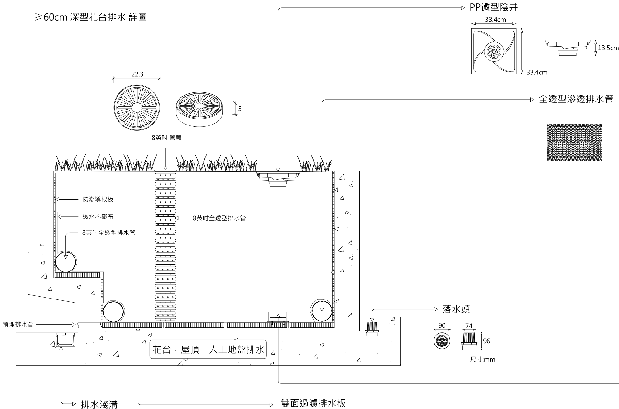
防潮阻根板
