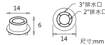
轉接頭腳座
