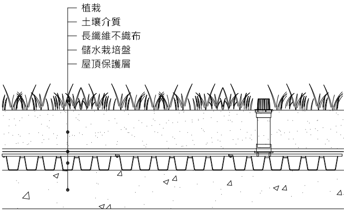
薄層綠屋頂儲水植栽盤詳圖
