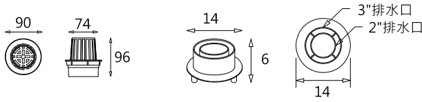
3英吋高平落水頭
