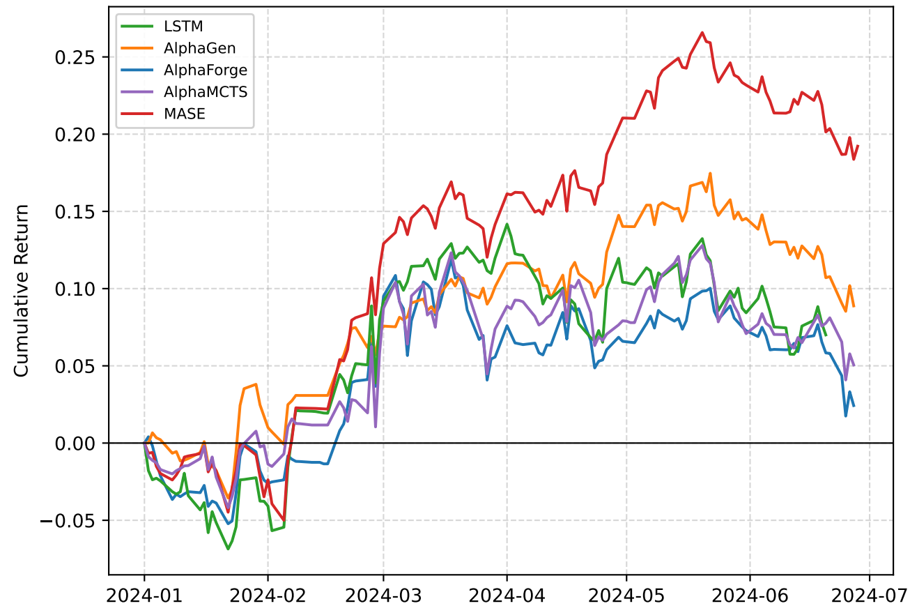
CSI300: 20240101-20240630
