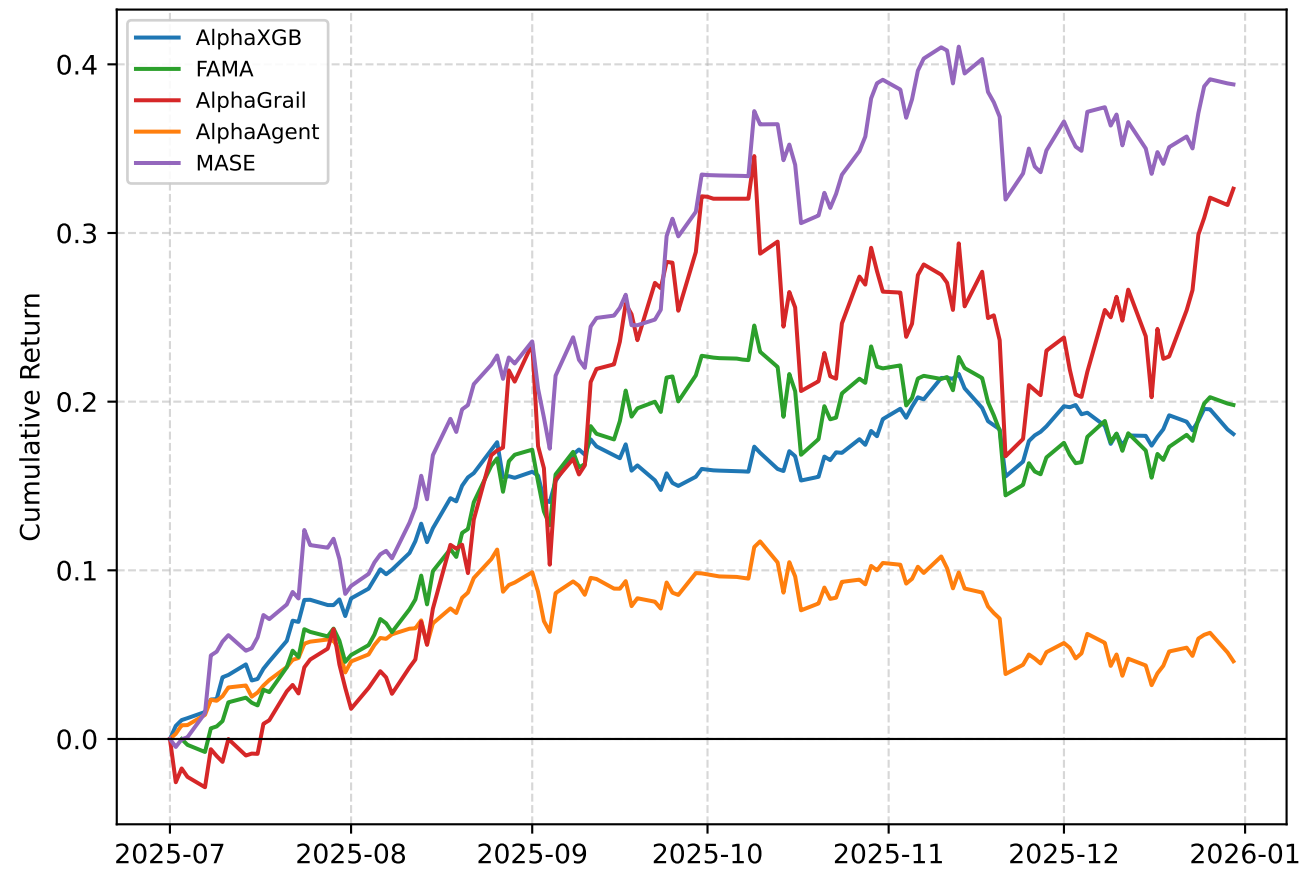
CSI500: 20250701-20251231
