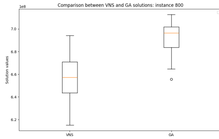
(d) I, J, K, E, S, Q, N1, N2, N3, M = 800
