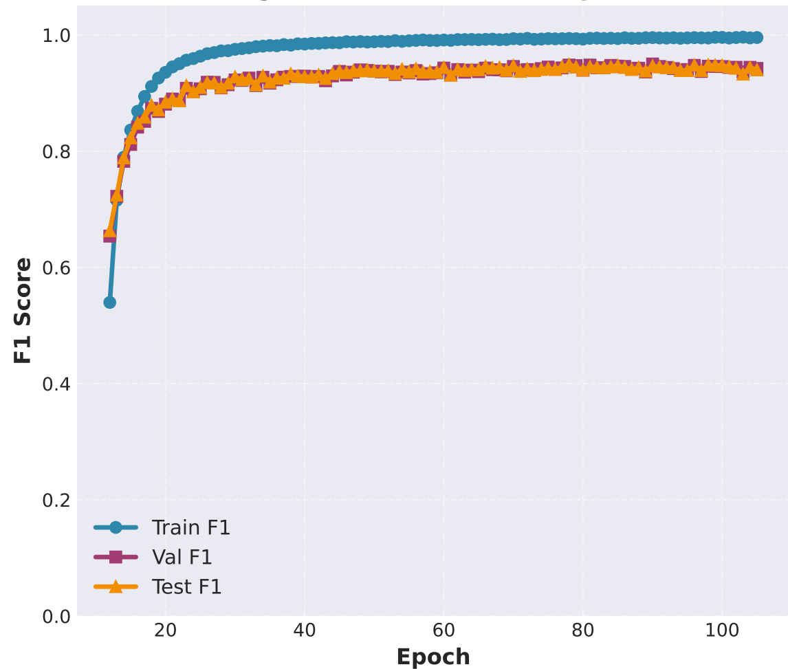
Weighted F1 Score Over Epochs
