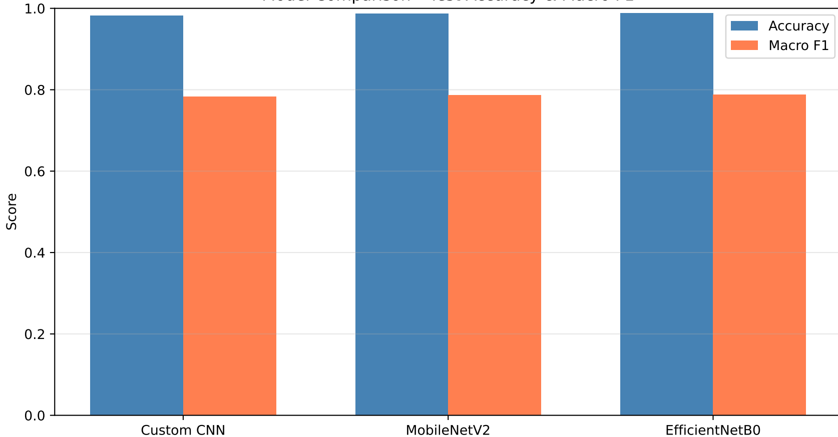
Model Comparison - Test Accuracy & Macro F1
