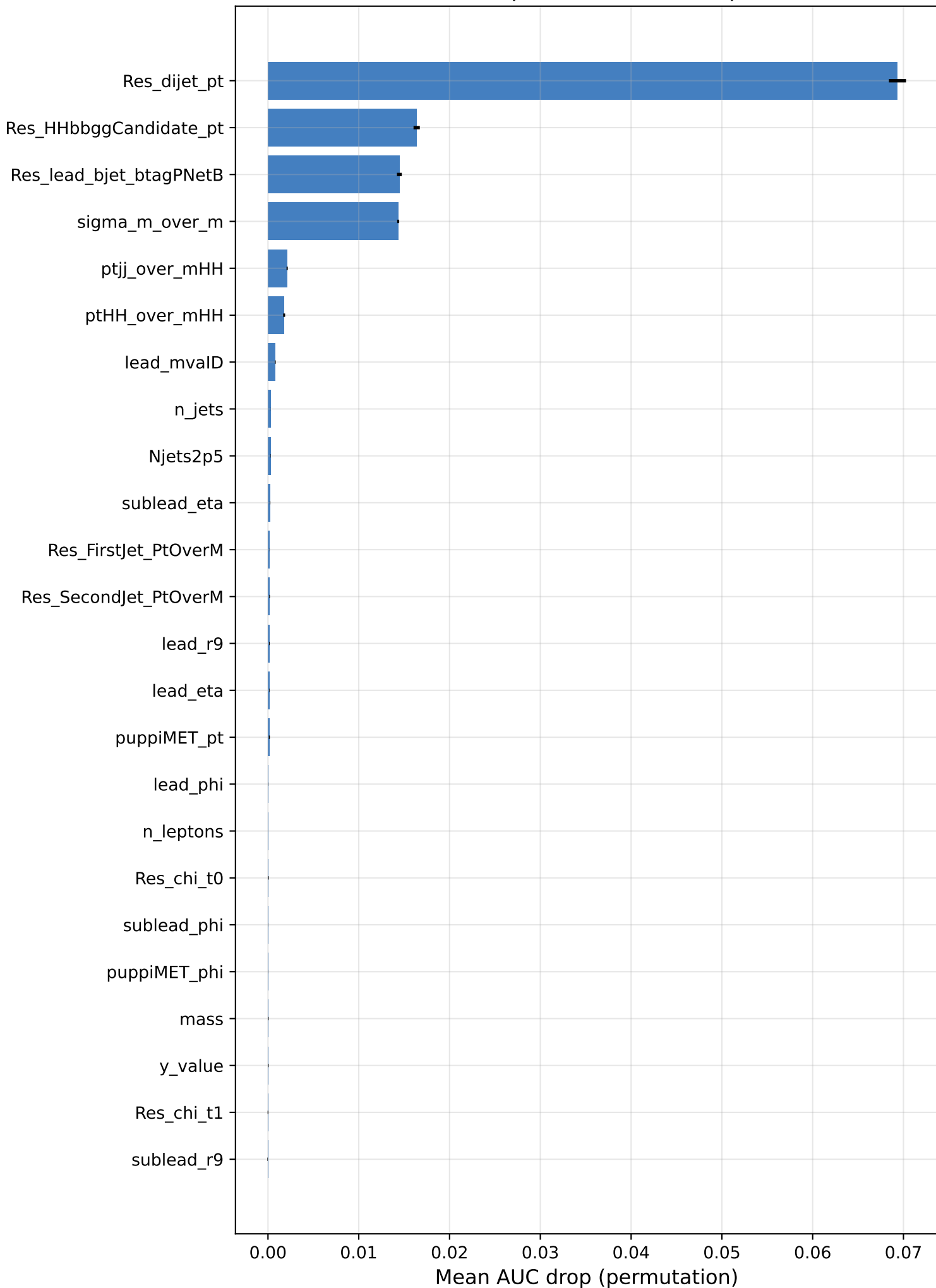
Permutation importance (AUC drop) -- TEST
