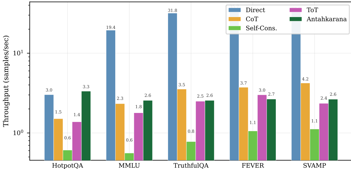
(d) Throughput Comparison Across Benchmarks
