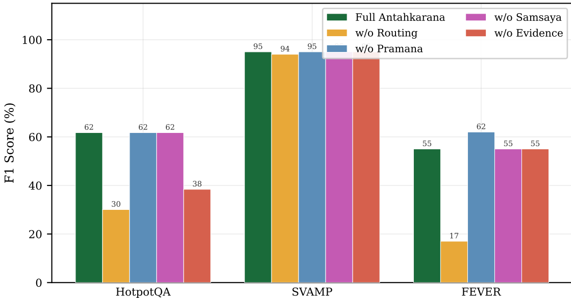
(e) Ablation Study — F1 Score
