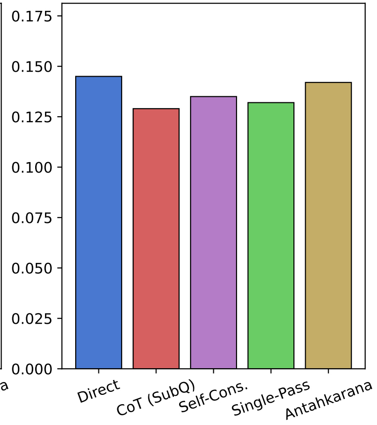
Macro-F1
