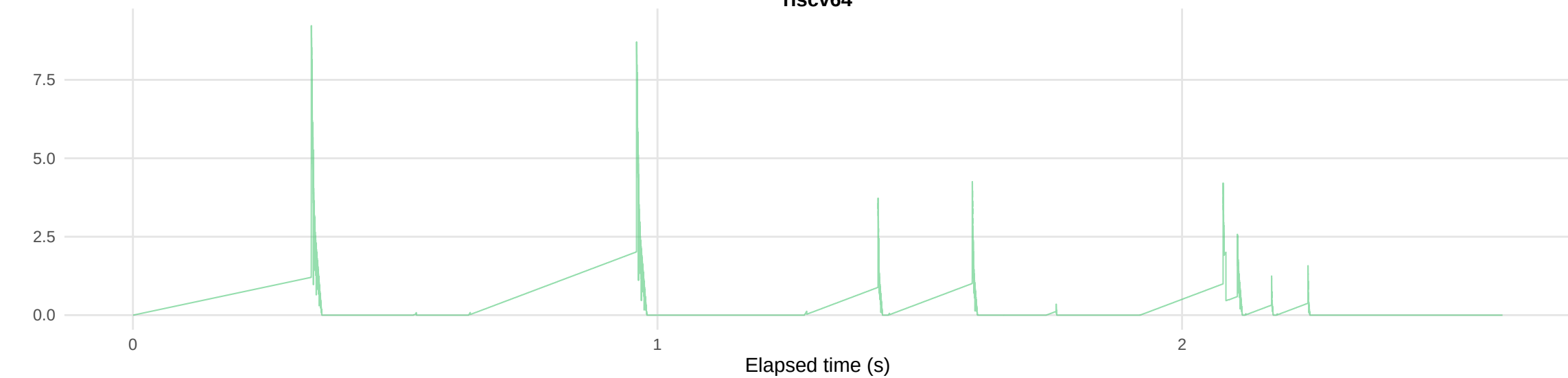
riscv64
