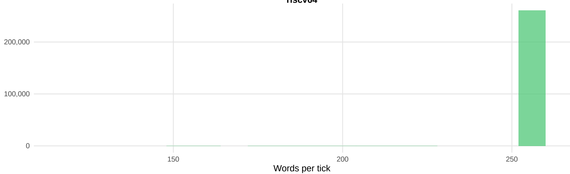
riscv64
