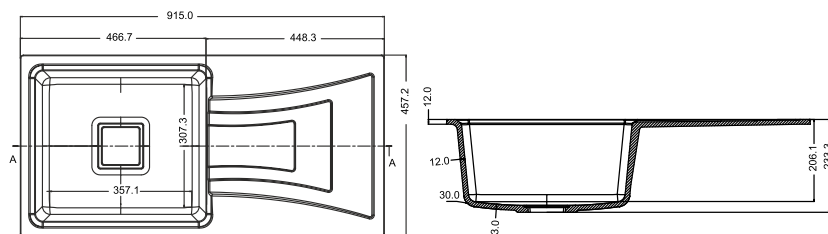
DIMENSIONS
