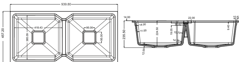
DIMENSIONS
