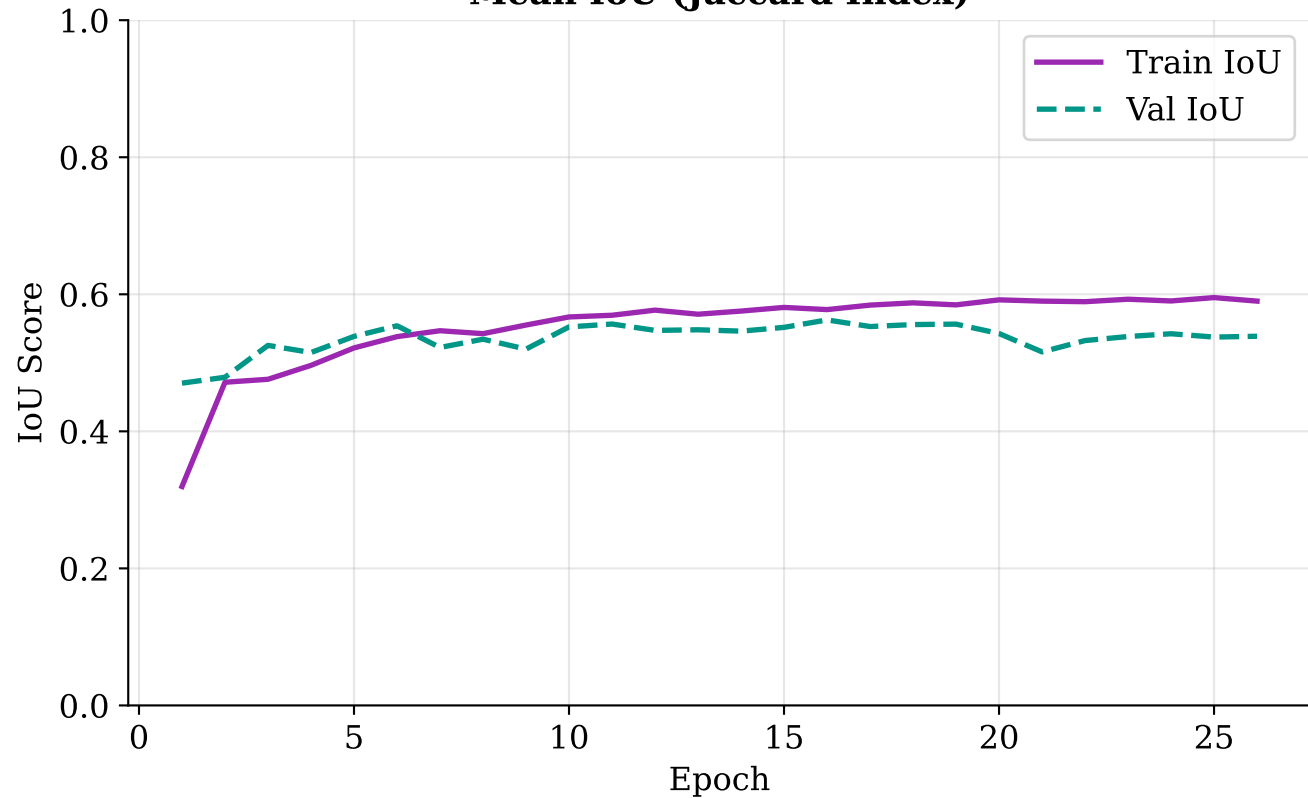
Mean IoU (Jaccard Index)
