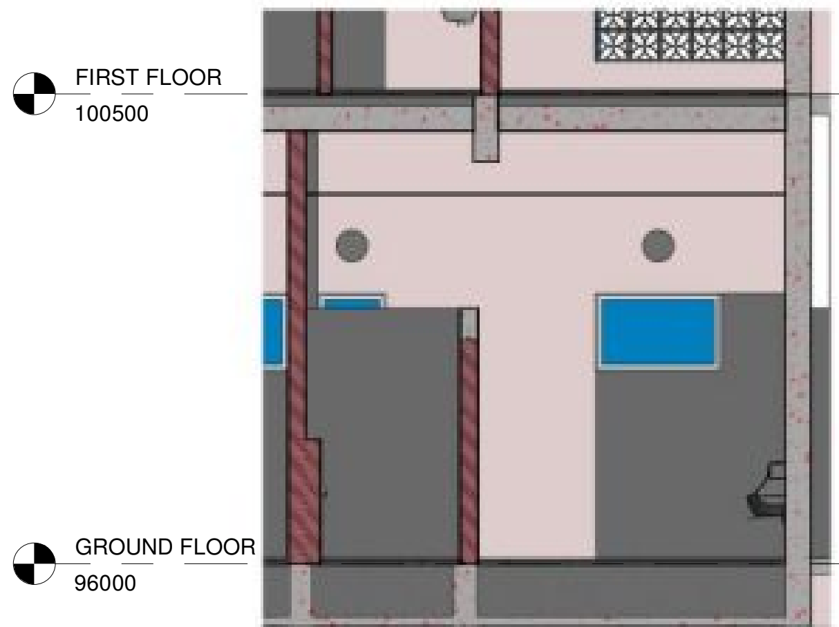
5 Elevation - 5 1 : 50
