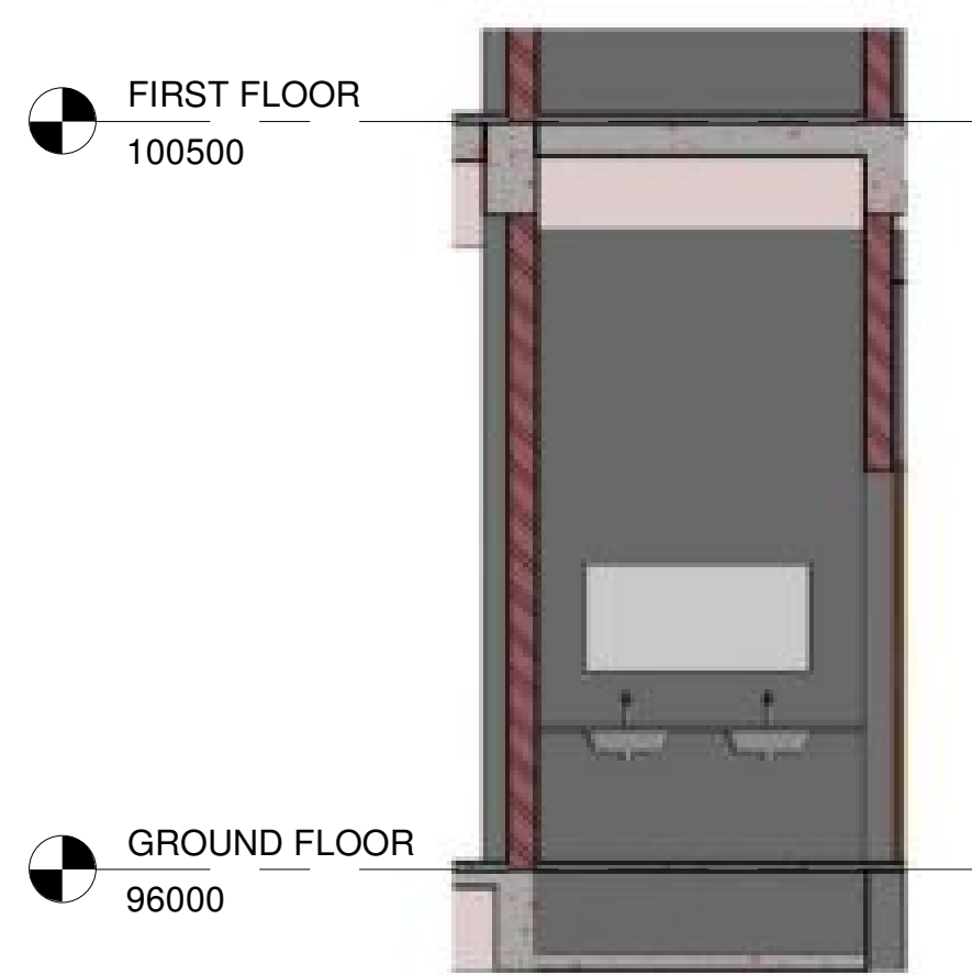
2 Elevation - 2 1 : 50
