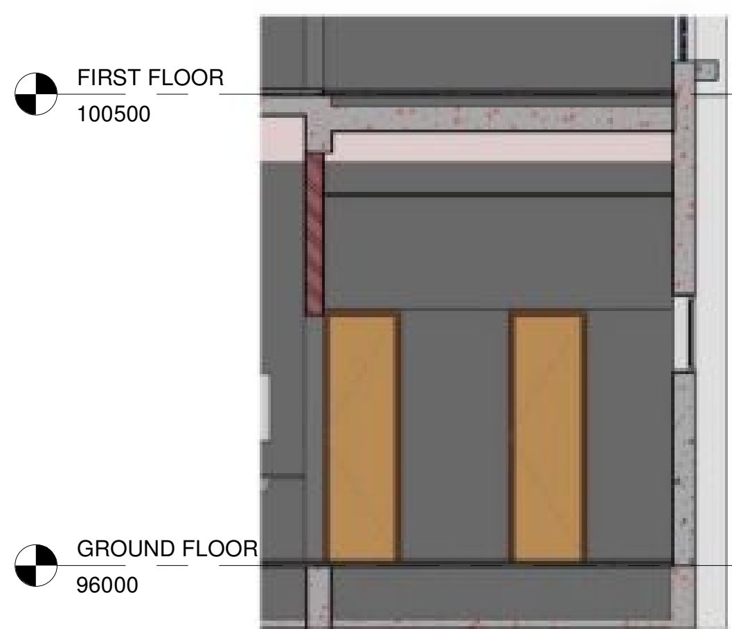
6 Elevation - 6 1 : 50
