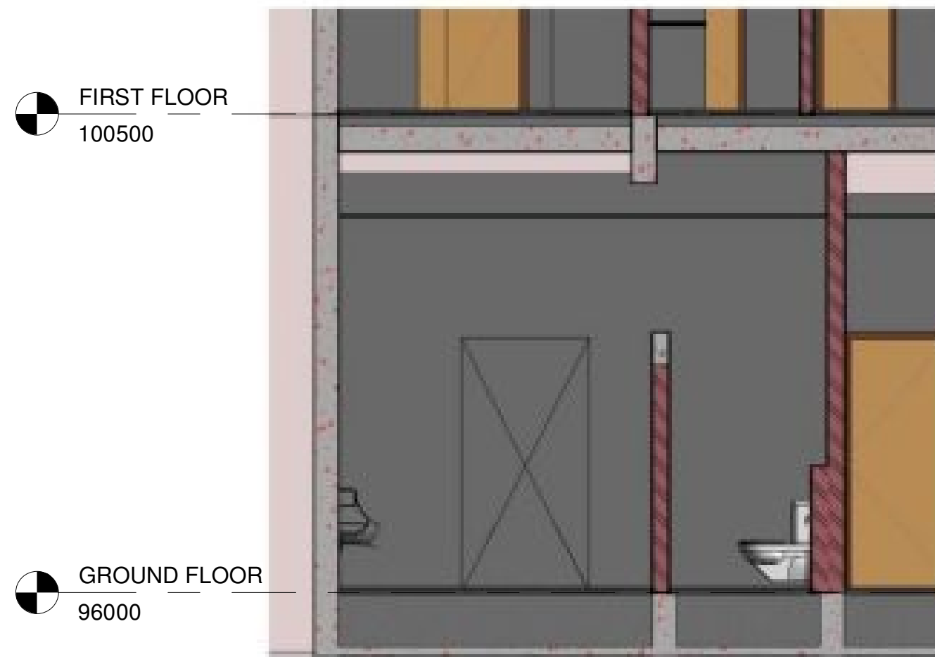
7 Elevation - 7 1 : 50
