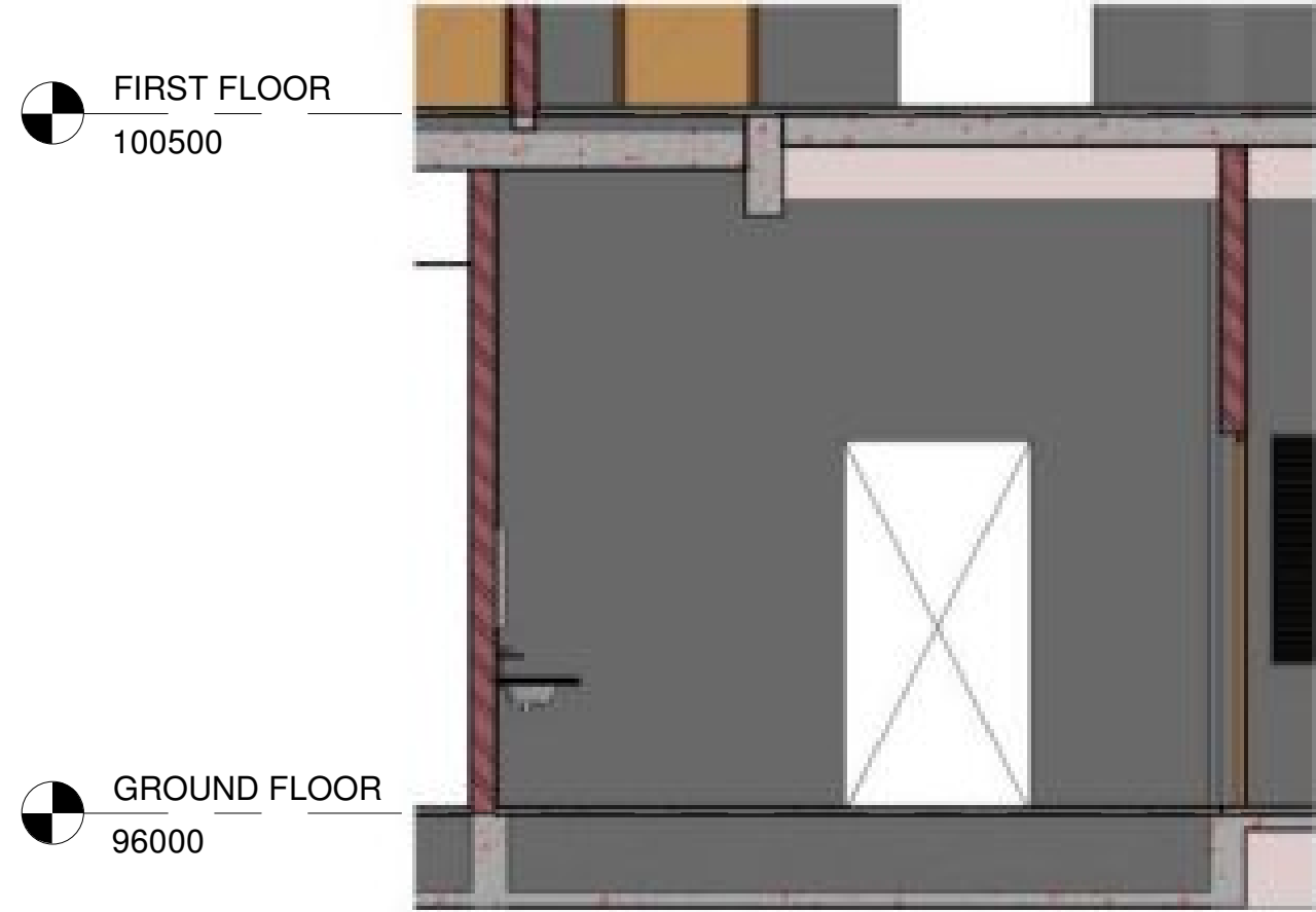
1 Elevation - 1 1 : 50
