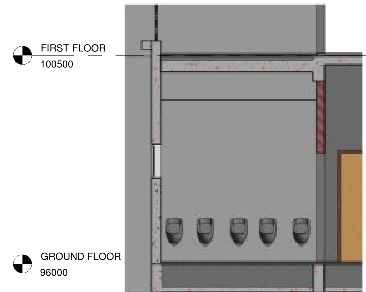
8 Elevation - 8 1 : 50
