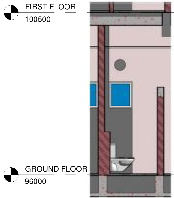
13 Elevation - 13 1 : 50
