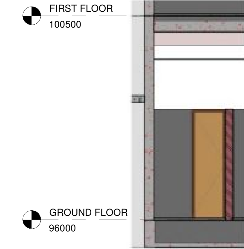
16 Elevation - 16 1 : 50
