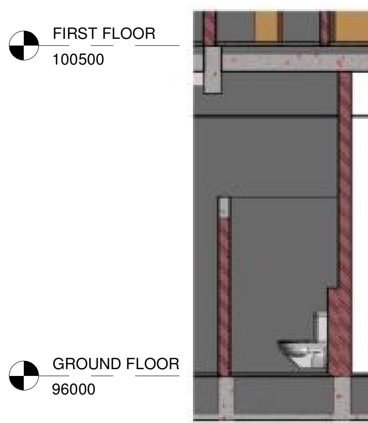
15 Elevation - 15 1 : 50
