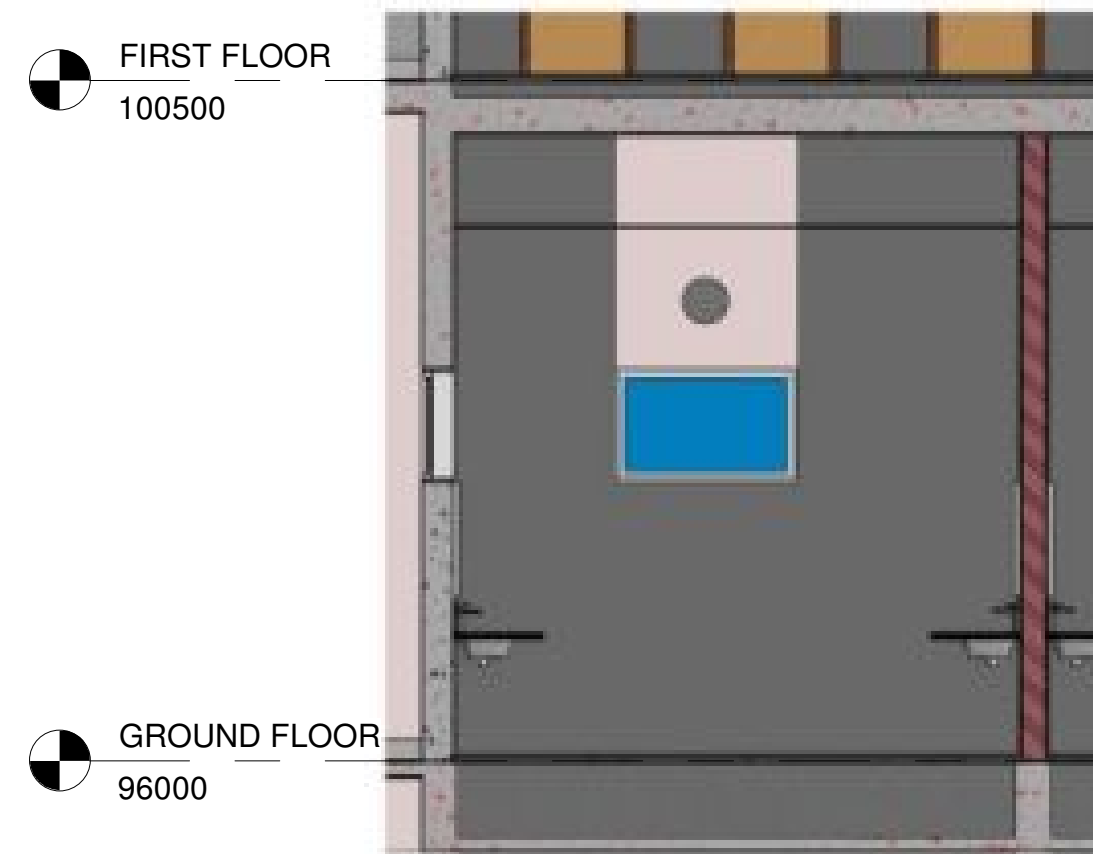
21 Elevation - 21 1 : 50
