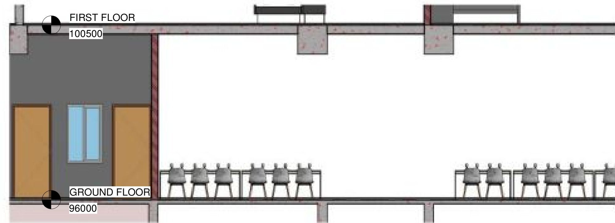
33 Elevation - 33 1 : 60
