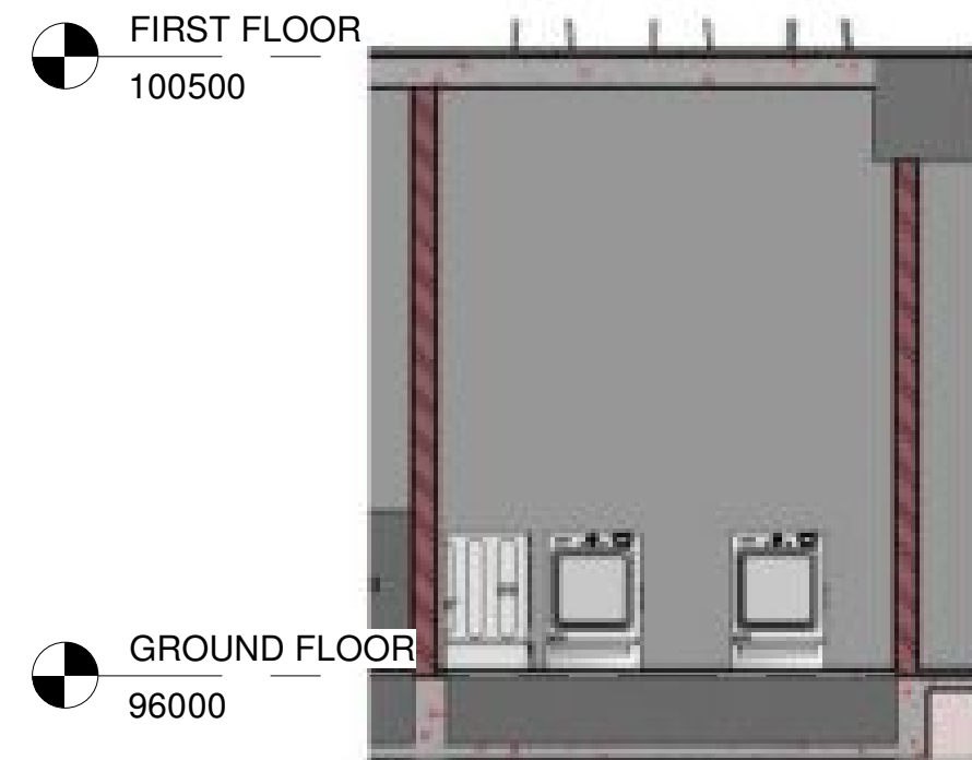
32 Elevation - 32 1 : 60
