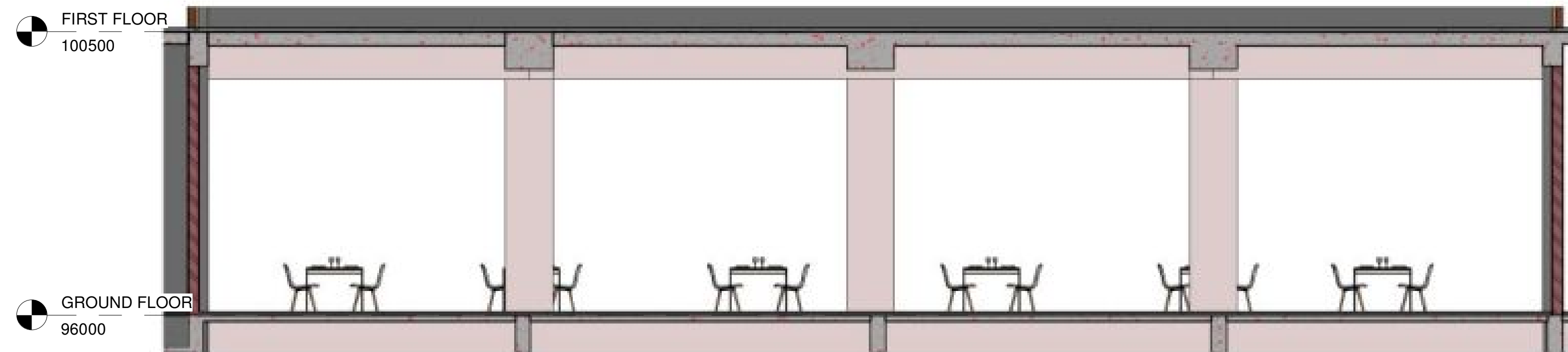
34 Elevation - 34 1 : 60
