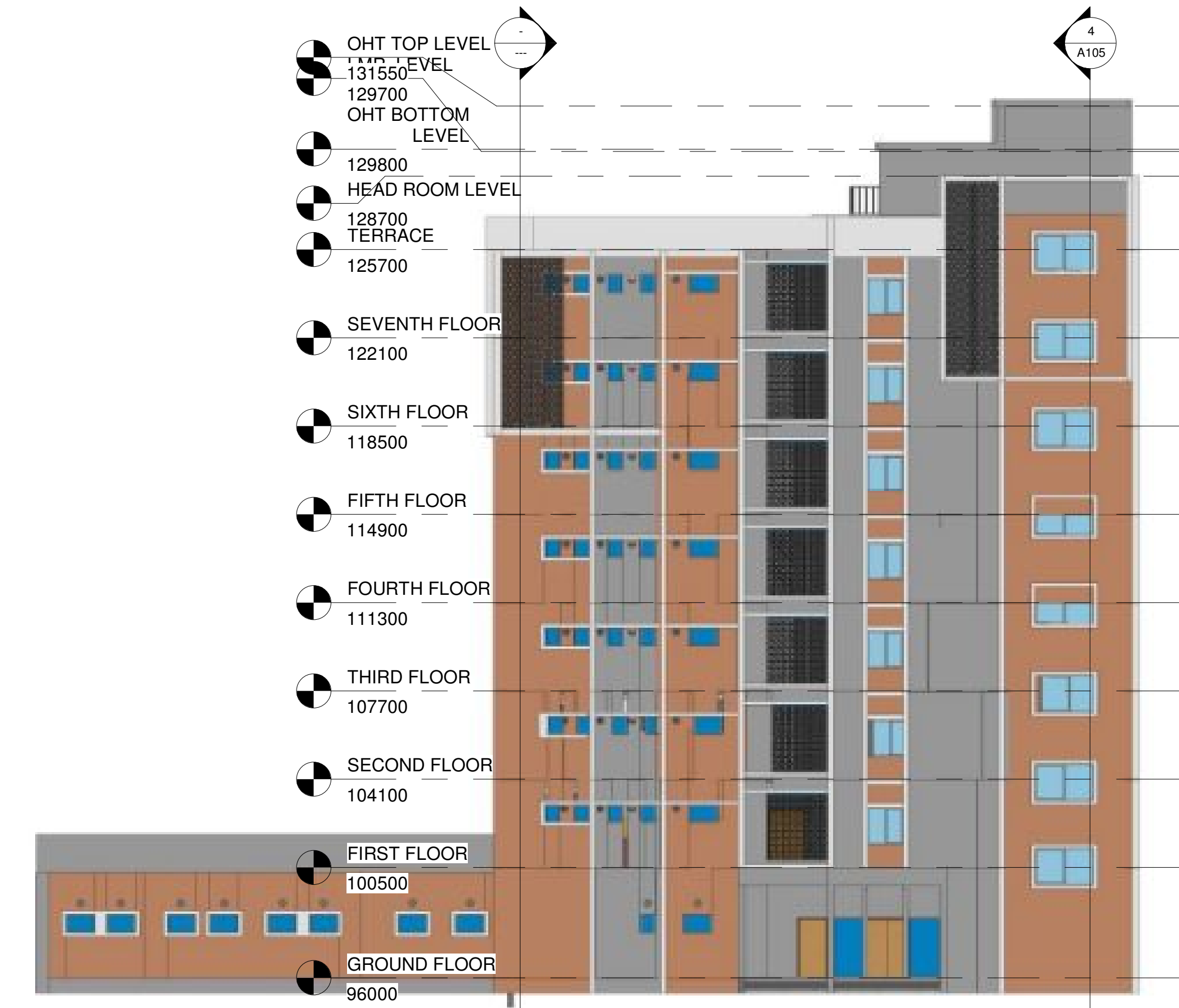
1 North 1 : 175
