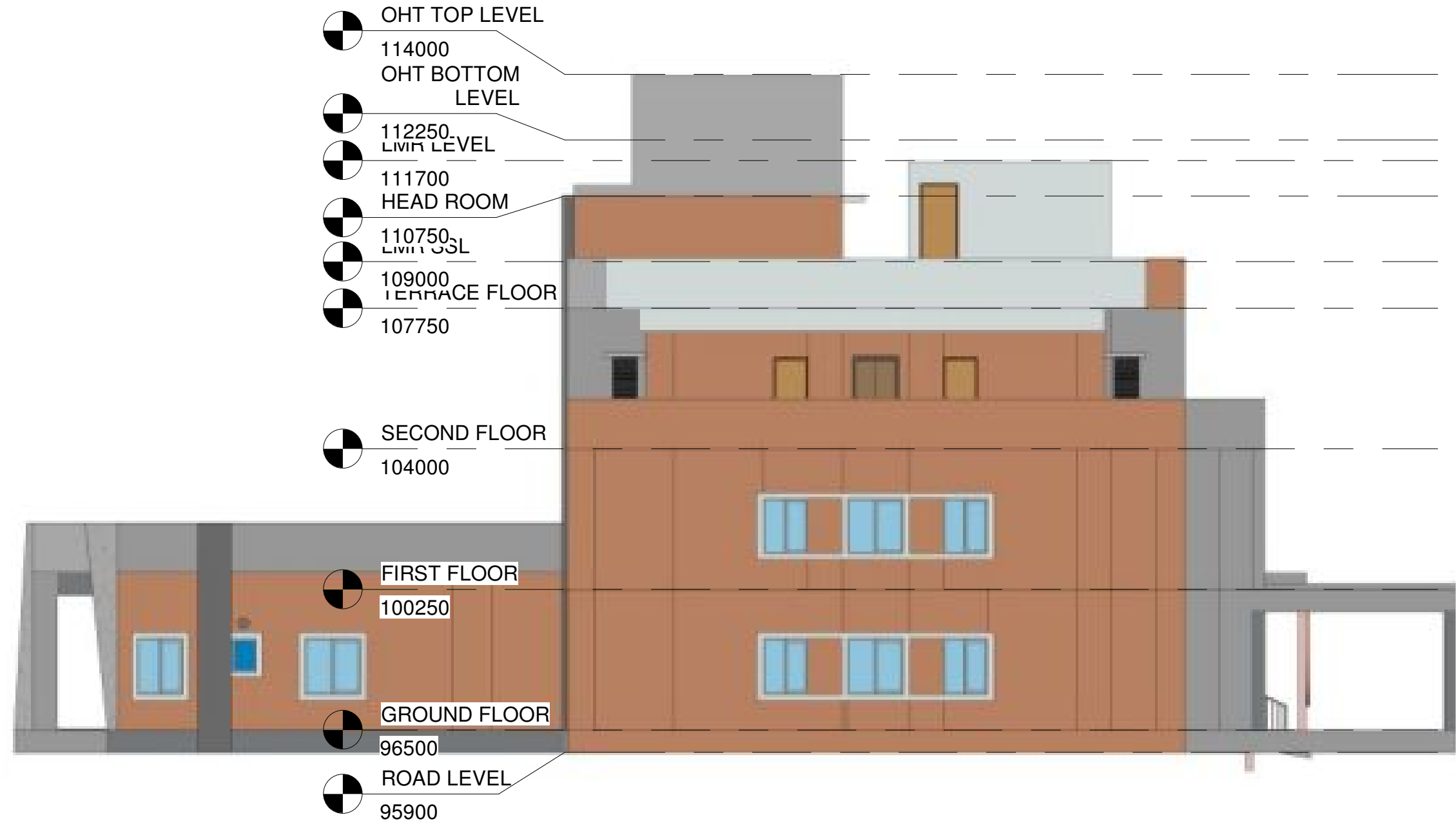
2 East 1 : 130
