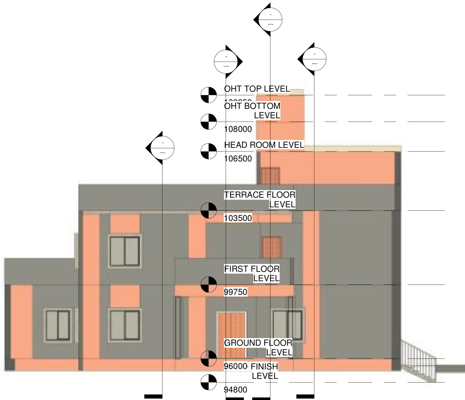
3 West 1 : 100
