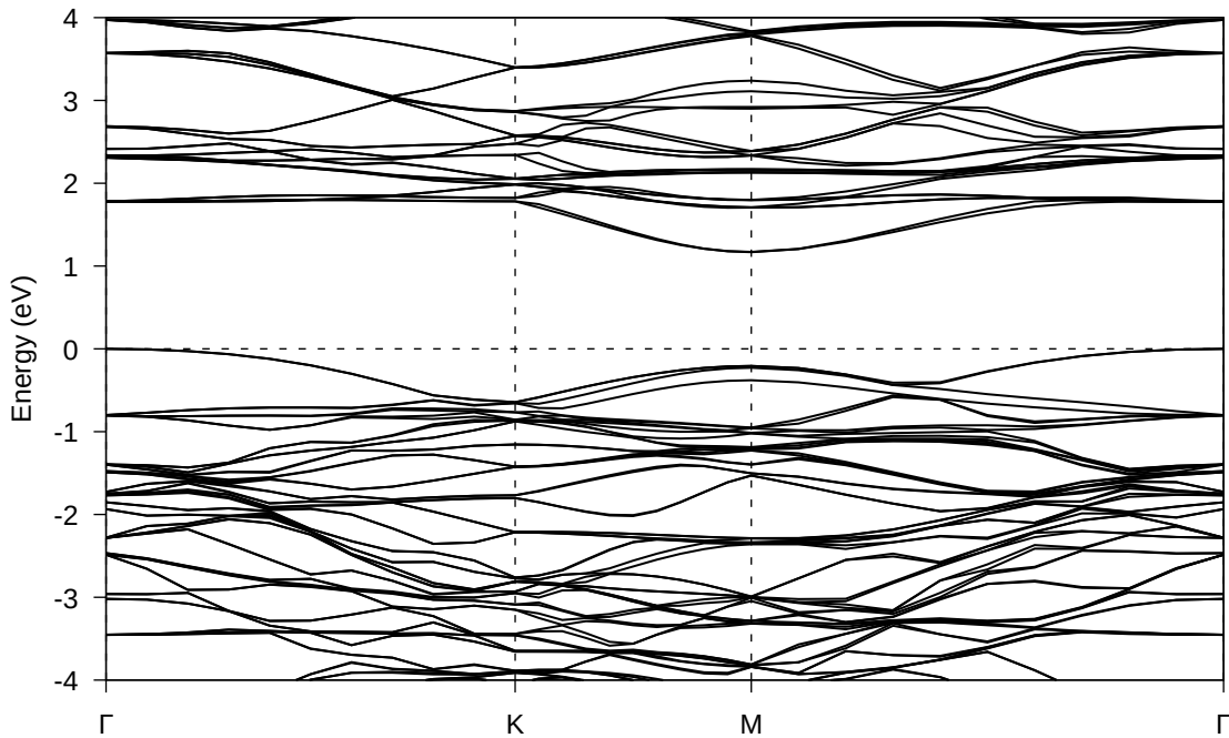
BN/MoS2 Bandstructure
