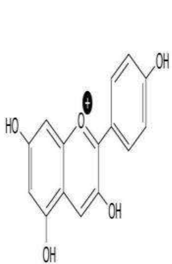
Pelargonidin
