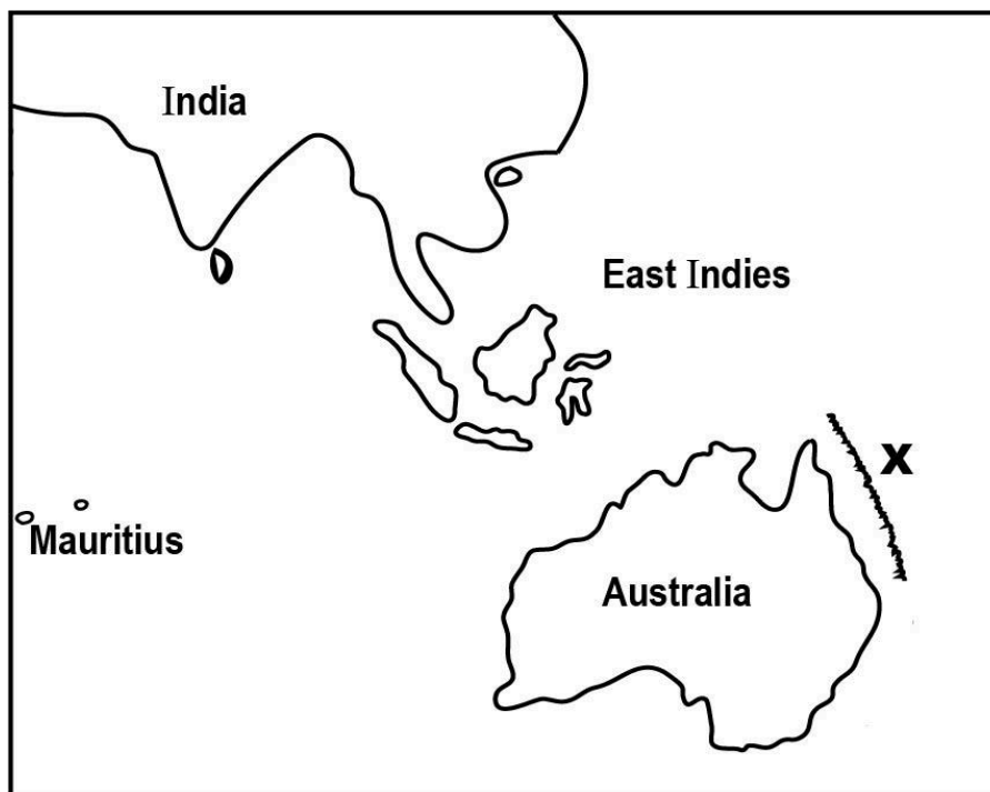
Map 2
