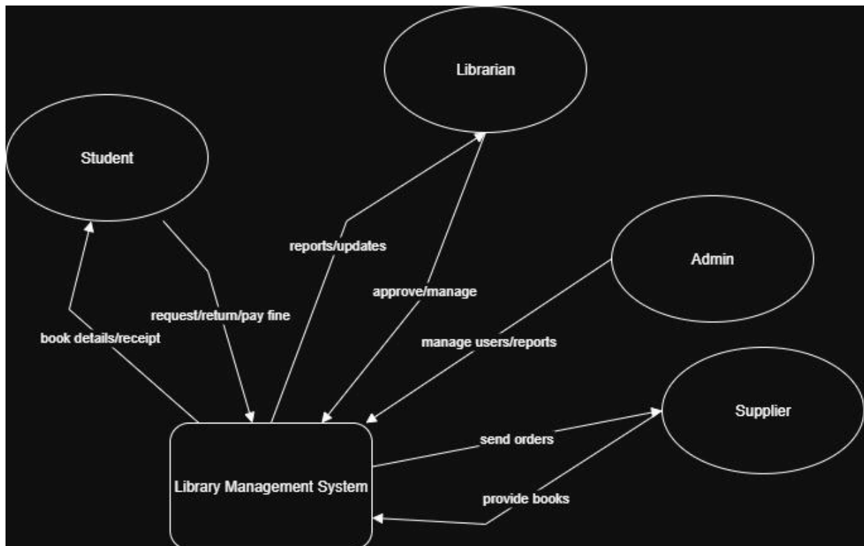
DFD Diagrams:
