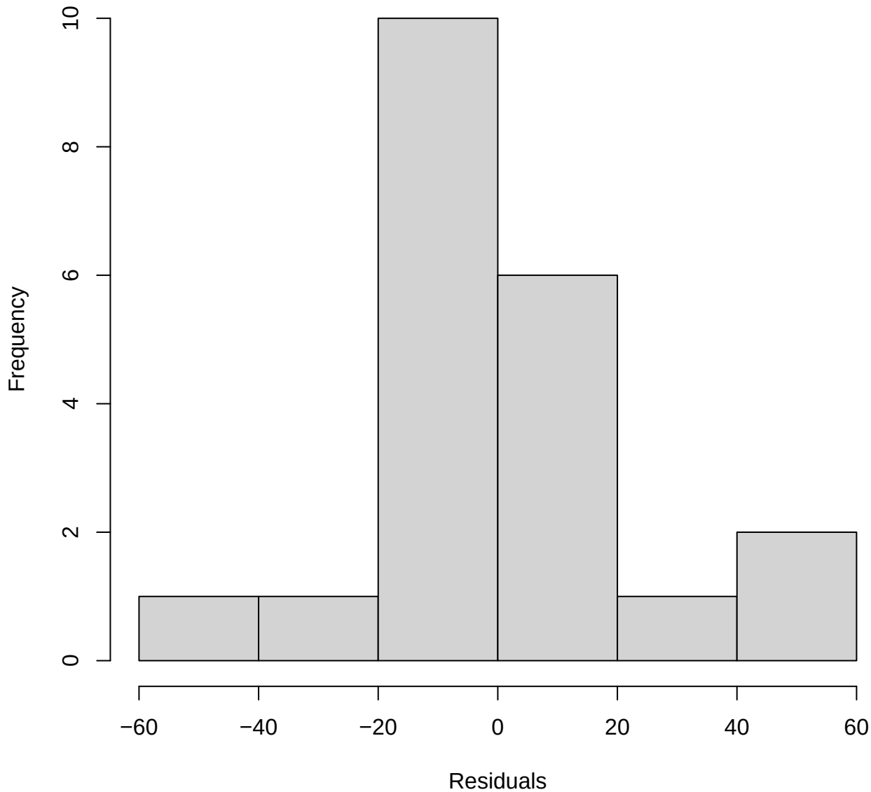
HW02 (d): Residuals Histogram
