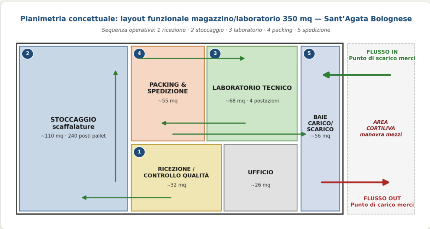
Fig. 11.1 — Planimetria concettuale: zone funzionali e sequenza operativa.
