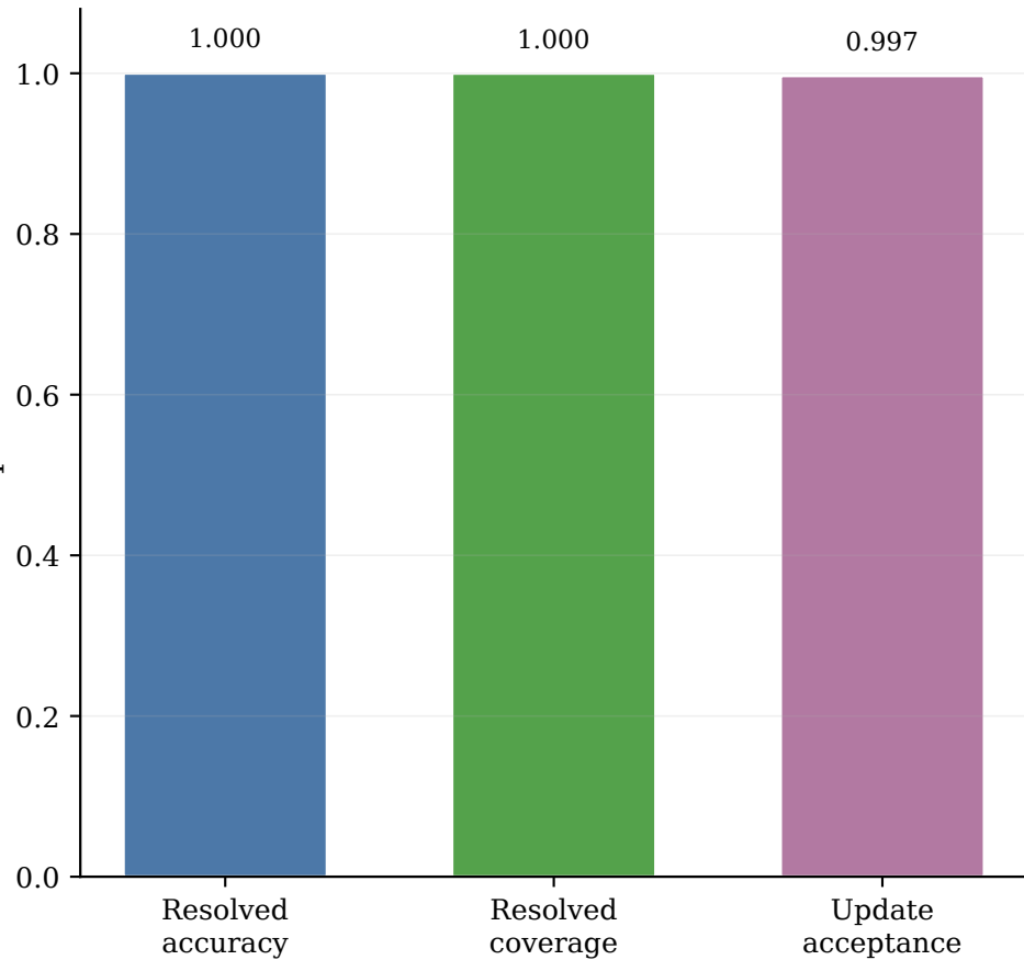
CartPole-v1
