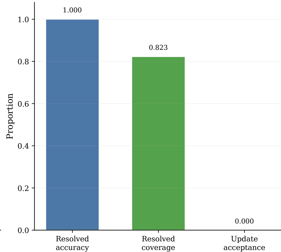
LunarLander-v3
