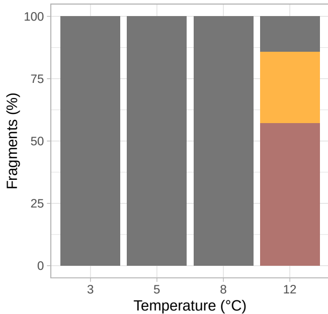
P.arborea
