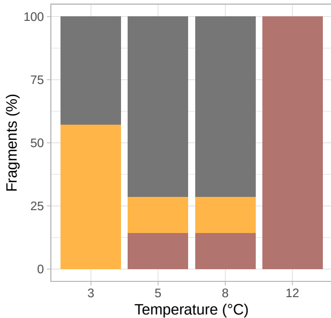
P.resedaeformis
