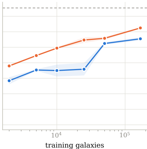
ViT-S/16
