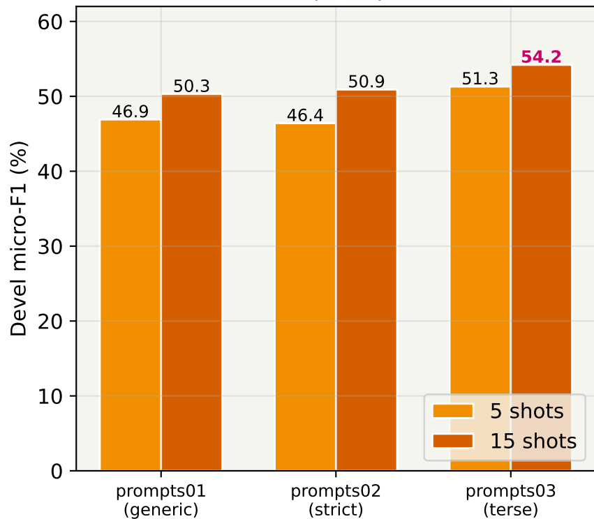
Micro-F1 — prompt × shots
