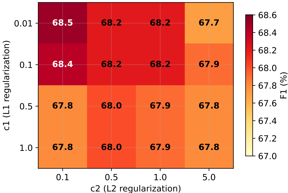
CRF Best F1 per (c1, c2) — mod6 Devel
