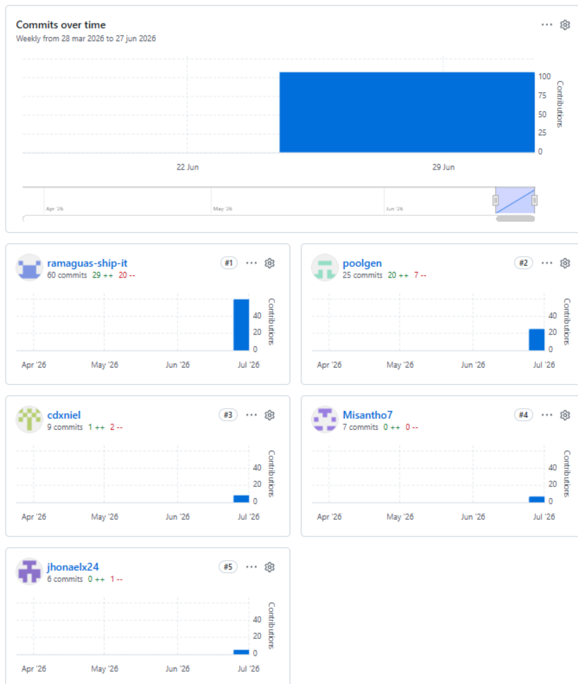
Ilustración 36. Commits
