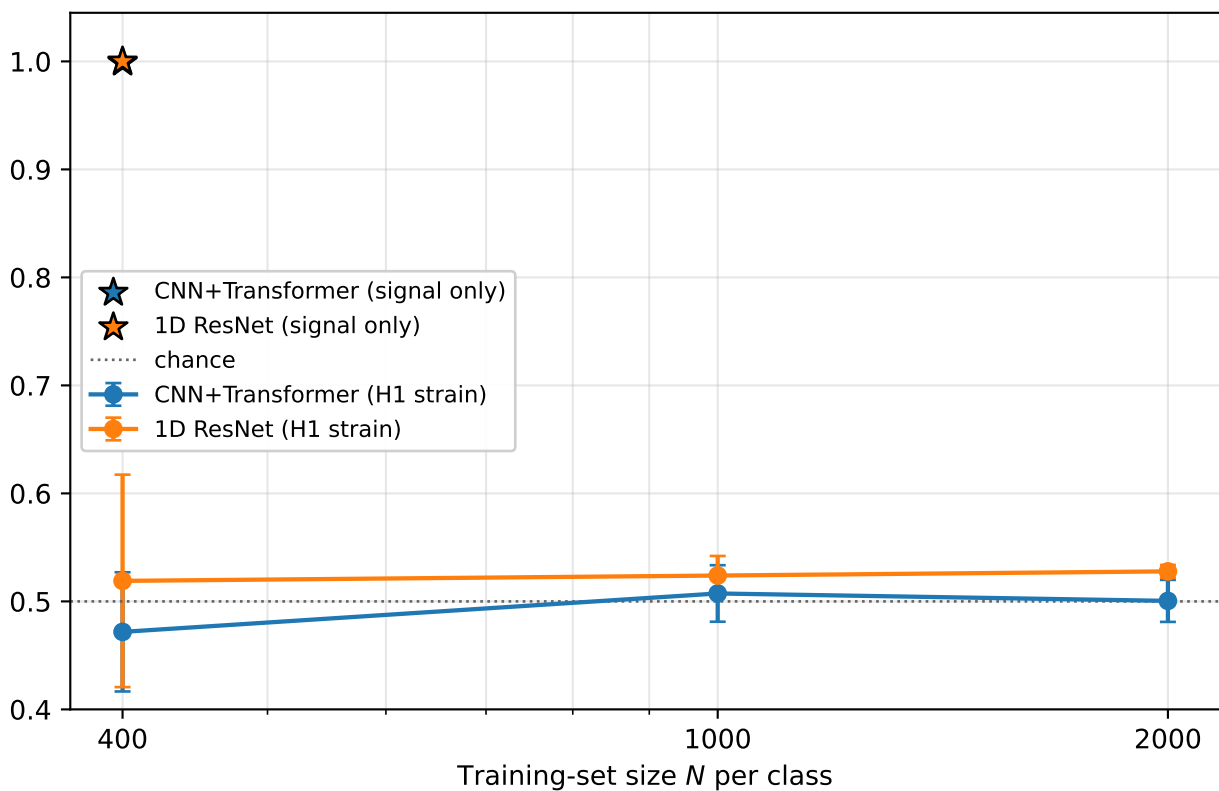
Best validation AUC
