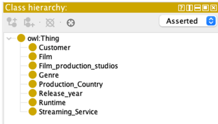
Figura 4-1: Classi dell'Ontologia
