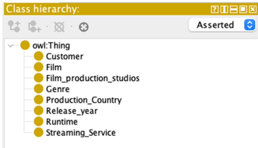
Figura 4-1: Classi dell'Ontologia
