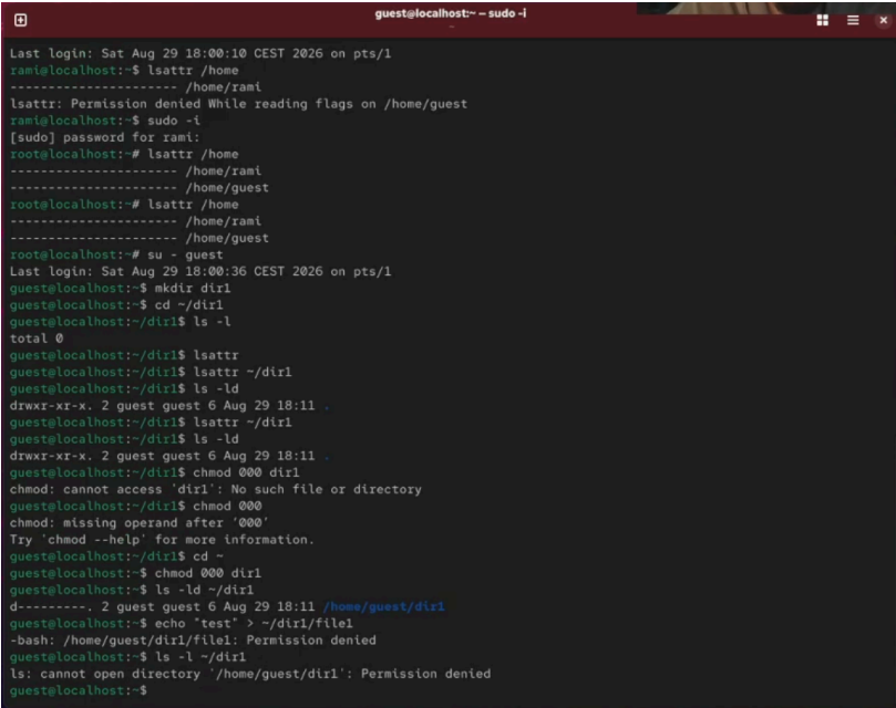
Рисунок 18. Проверка содержимого директории dir1
