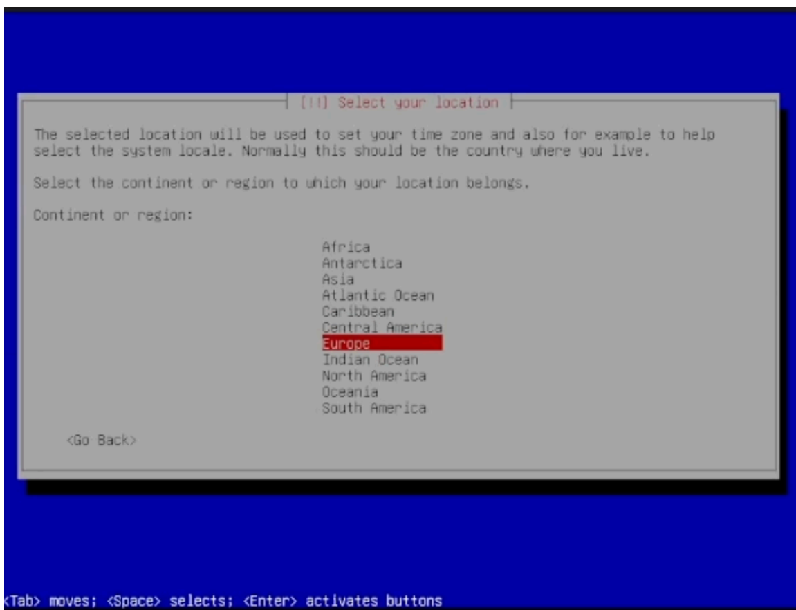
Рисунок 6. Локация
