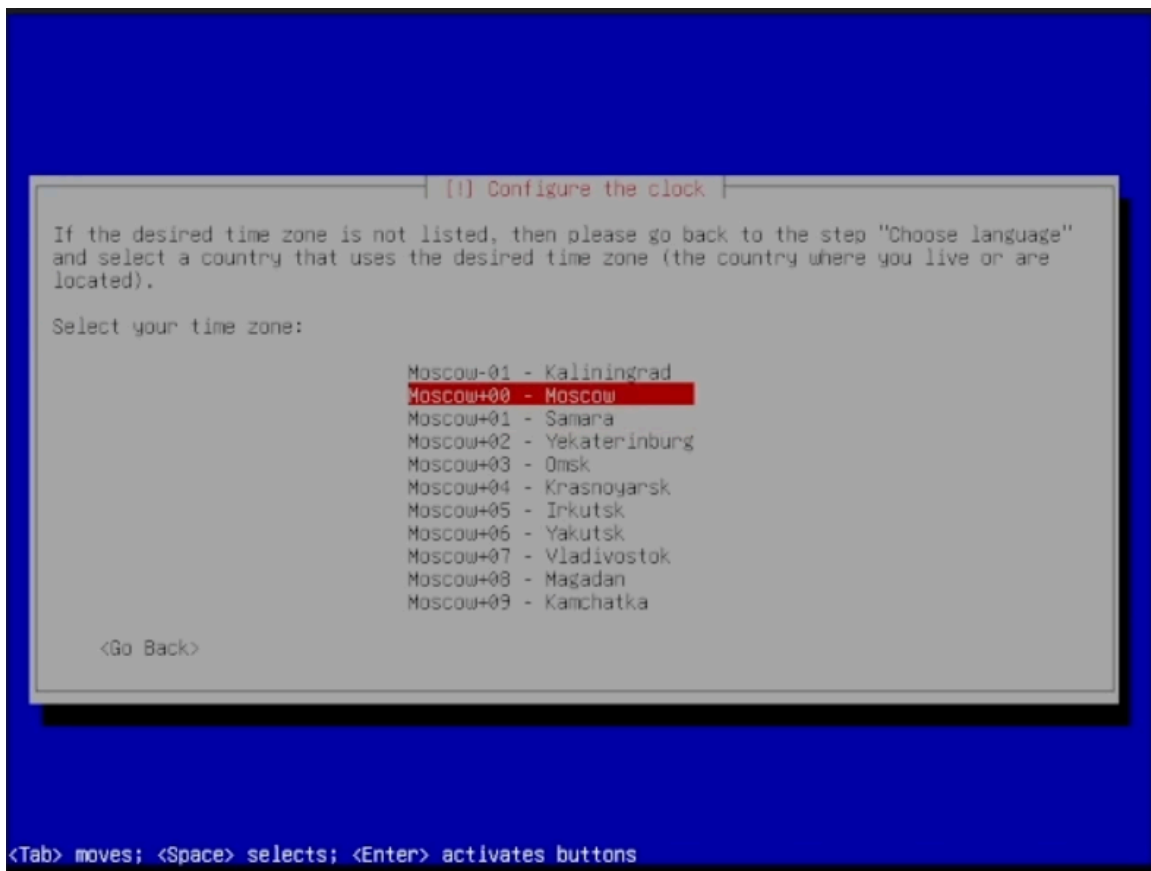
Рисунок 11. Настройки часов
