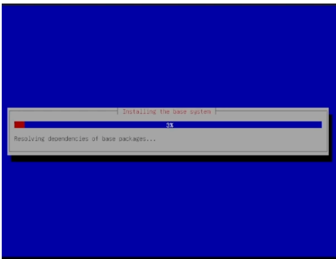
Рисунок 13. Установка системы
