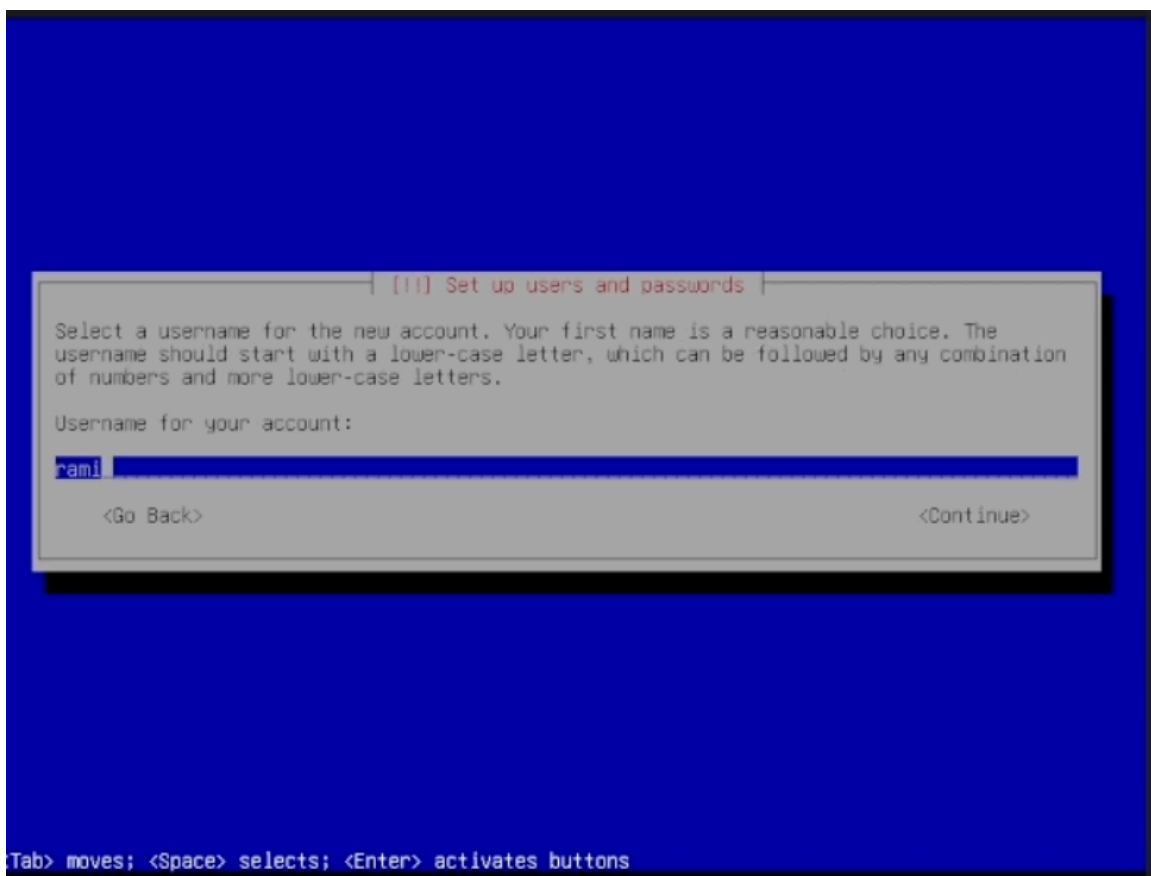
Рисунок 9. Создание пользователя
