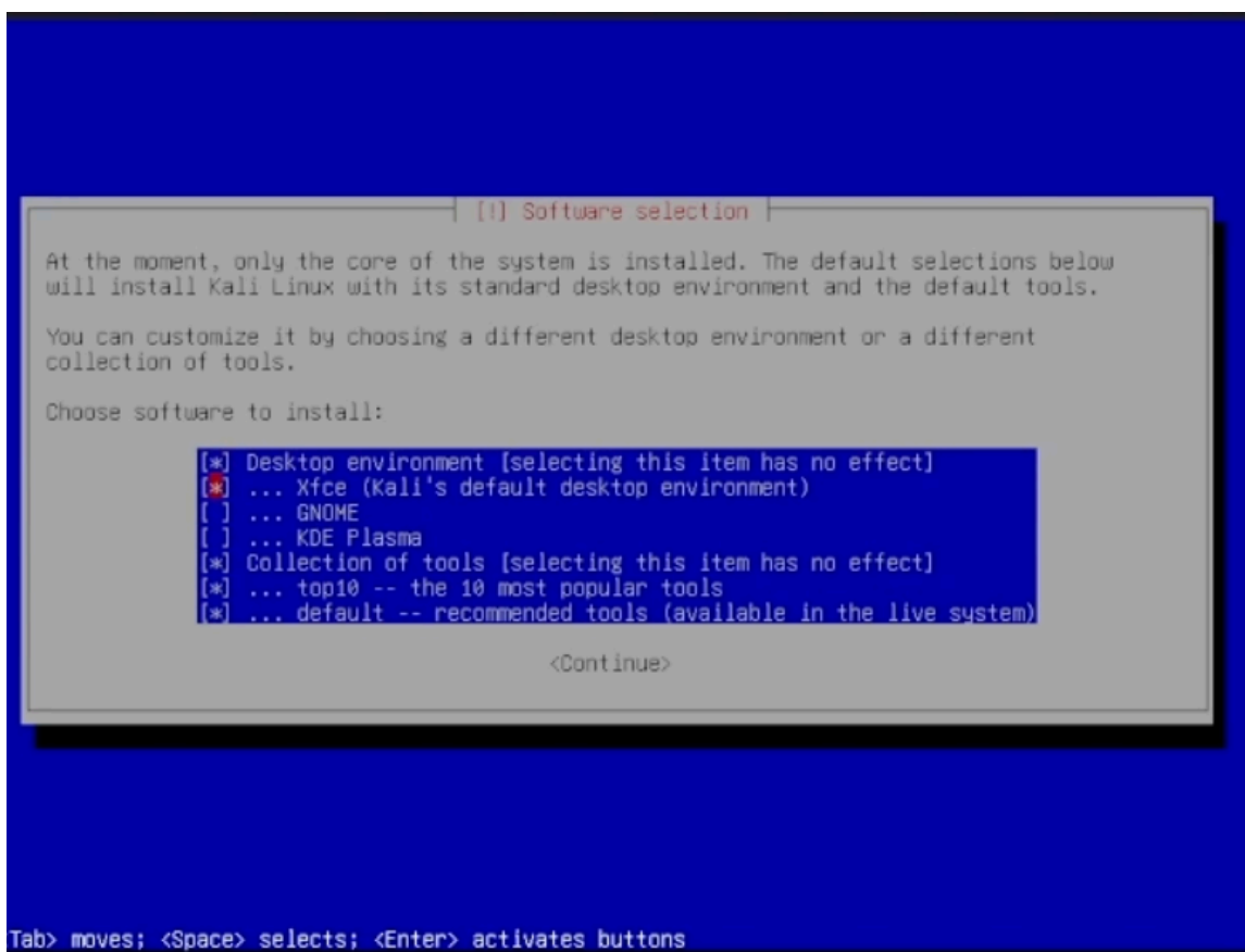
Рисунок 14. Выбор UI
