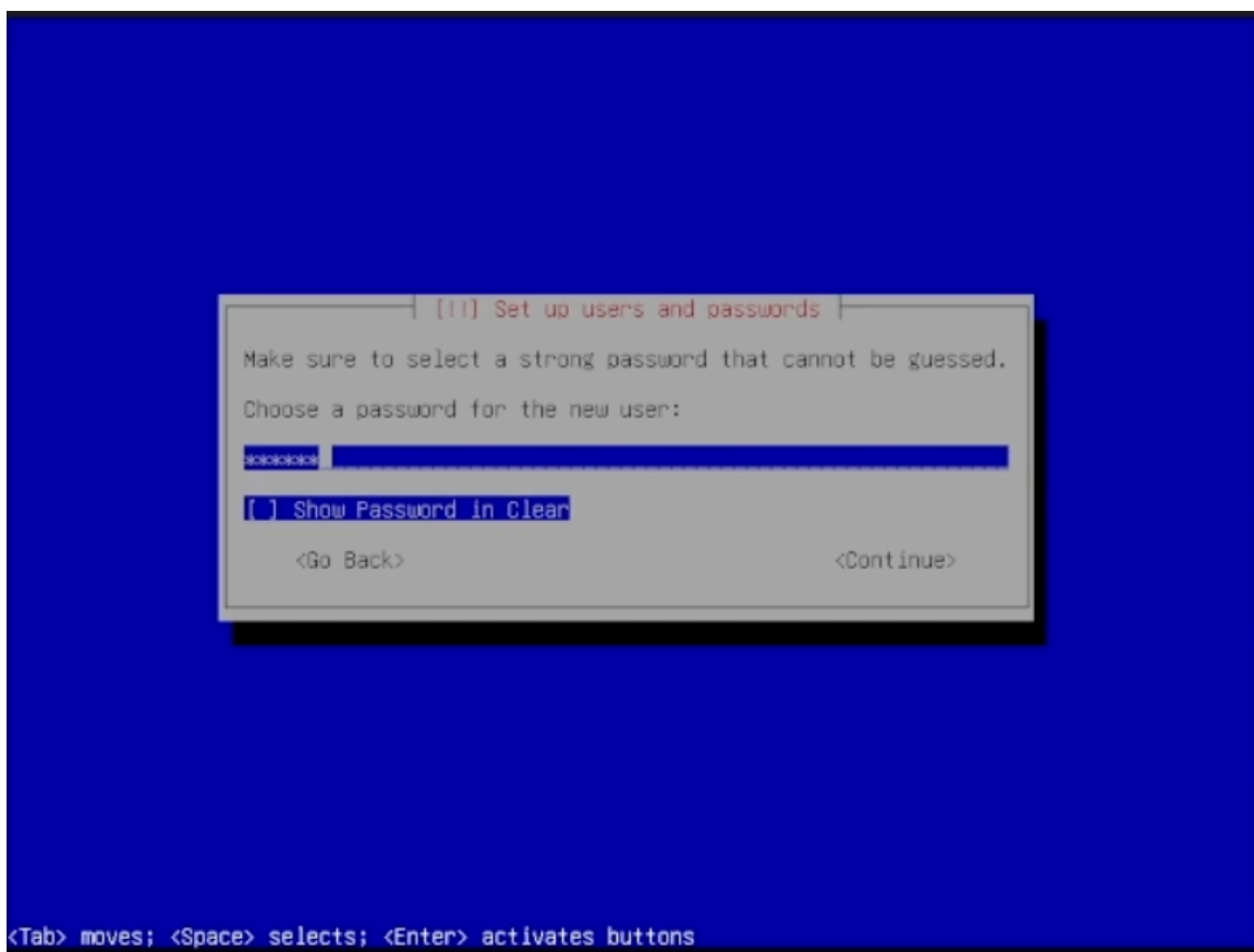
Рисунок 10. Установка пароля
