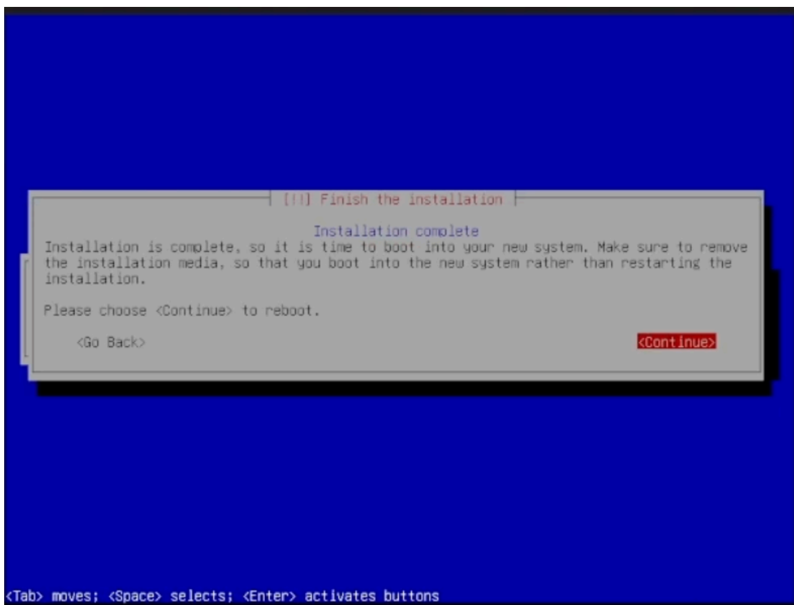
Рисунок 15. Завершение установки
