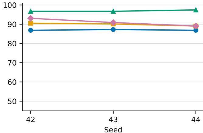
Qwen3-1.7B
