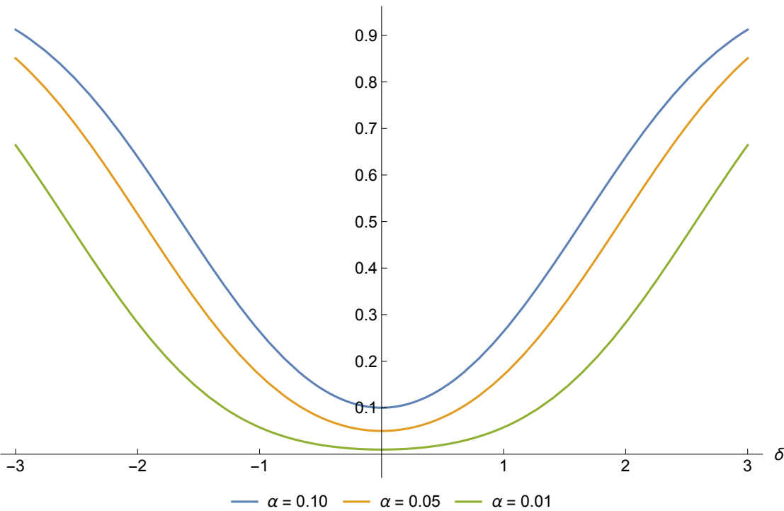
Poder asintótico local
