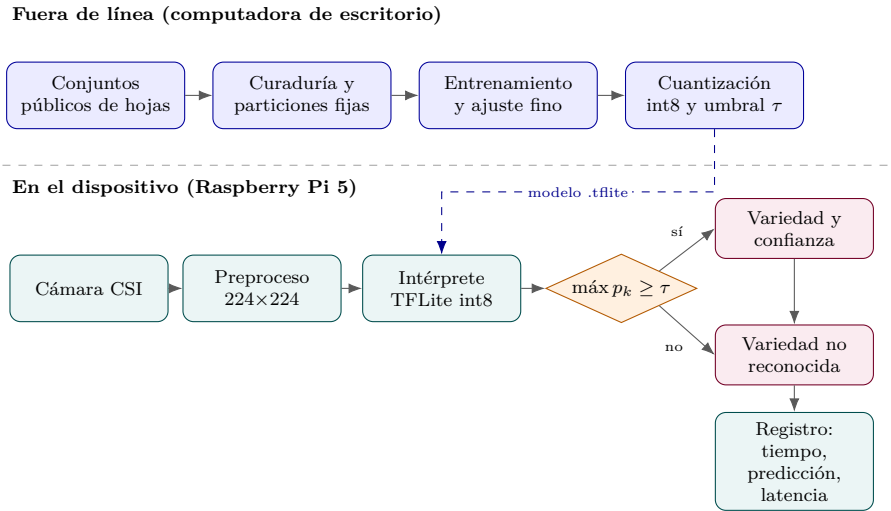
Figura 3.2: Arquitectura general del sistema: flujo de preparación del modelo fuera de línea y flujo de inferencia en el dispositivo.
