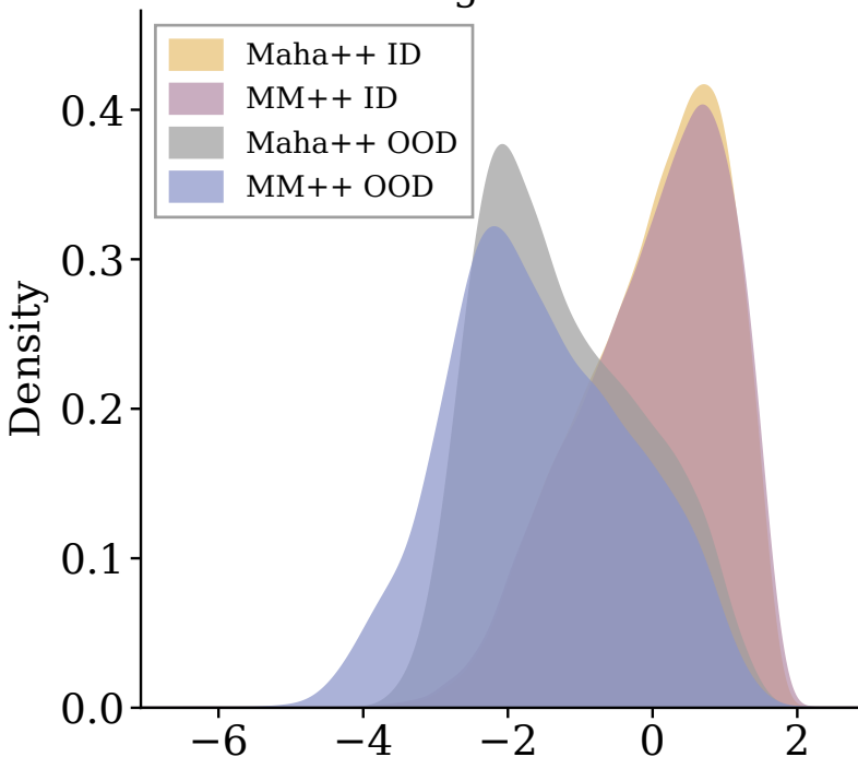
ImageNet-C
