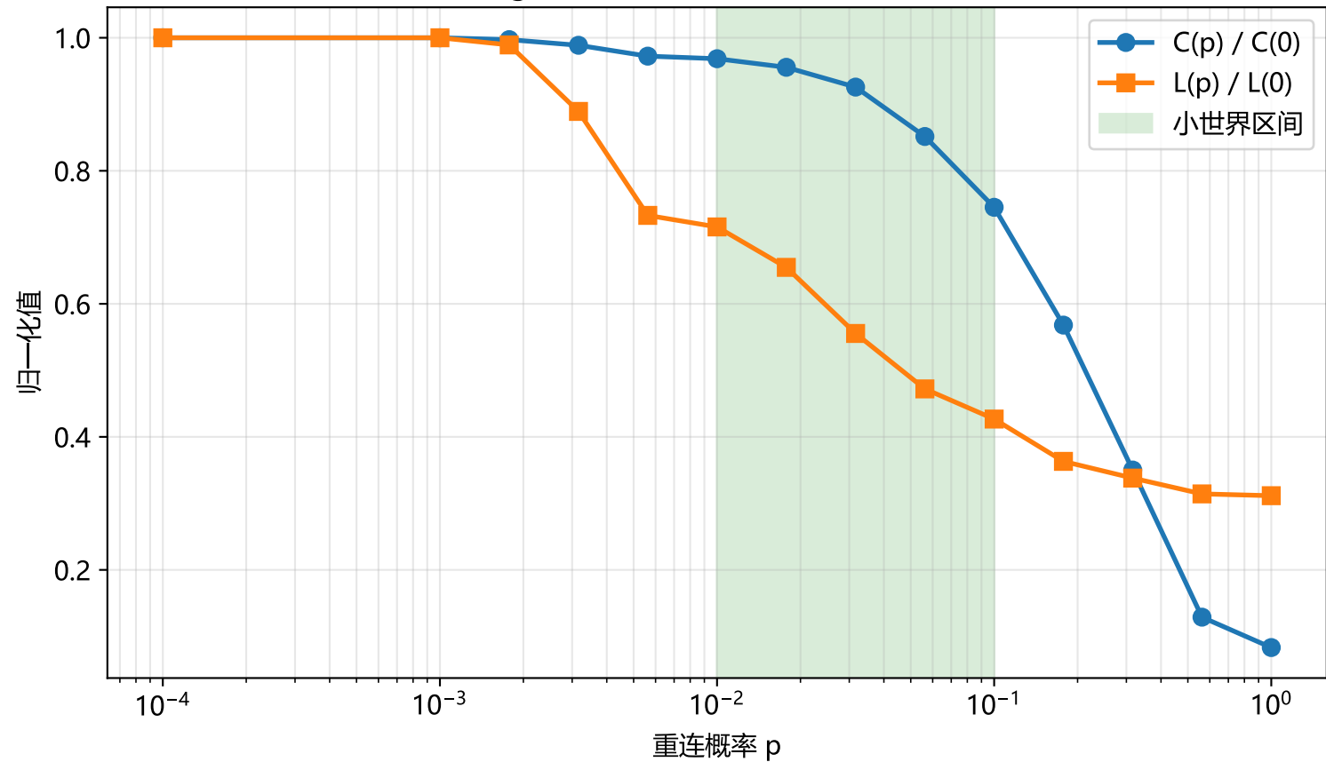
Watts-Strogatz 小世界特性 ( n=100, k=6, 5 次重复)
