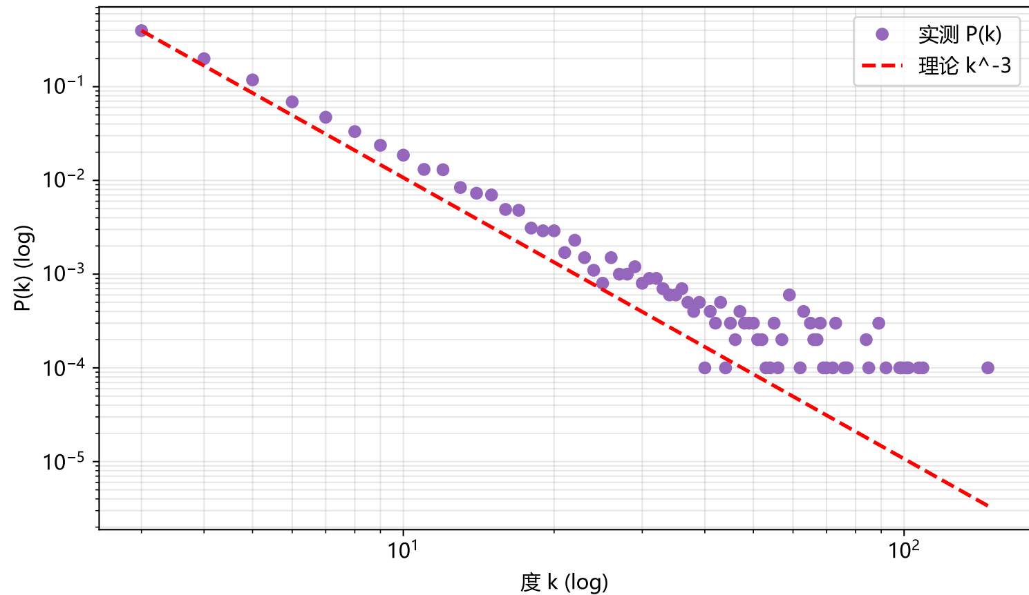
BA 模型度分布 (n=1000, m=3, 10 次合并)
